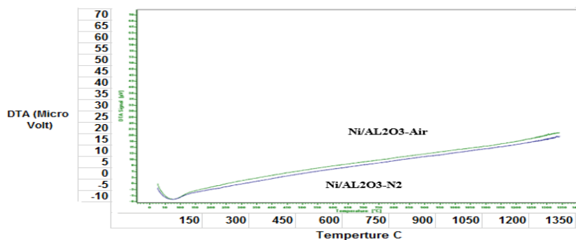
شکل ۹. پدیده‌های حرارتی کاتالیست نیکل بر پایه گاما آلومینا با آنالیز DTA.
