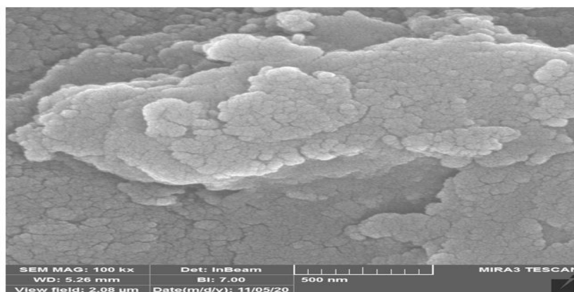
شکل ۶. ساختار ظاهری کاتالیست آلومینا با روش SEM و مقیاس ۵۰۰ nm.
