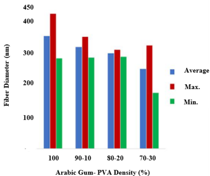
شکل ۵. بررسی تأثیر نسبت ضمغ عربی از صفر تا ۳۰ درصد بر متوسط اندازه قطر الیاف.
