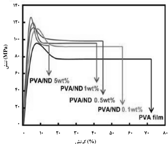
شکل ۱۰. نمودار تنش- کرنش پلی وینیل الکل و نانوذرات چندانسانه‌های آن با نانوذرات الماس [۲۵].
