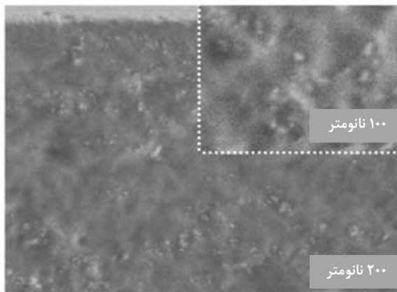
شکل ۱۱. تصویر میکروسکوپ الکترونی از سطح شکست نانوذرات چندانسانه ۵٪ وزنی پلی وینیل الکل با نانوذرات الماس [۲۵].
