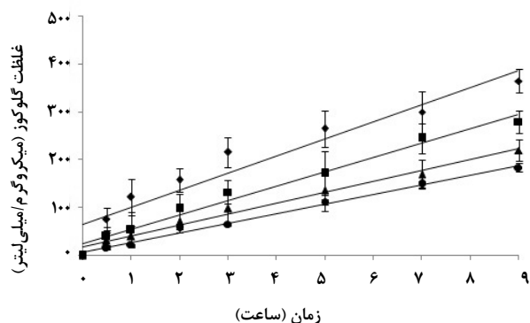
شکل ۶- غلظت گلوکوز به دست آمده از ۹ ساعت اولیه تخریب با آنزیم آلفا آمیلاز در دمای (25 \pm 1)^\circ\text{C} (◆) (نشاسته/ پلی وینیل الکل) / ۱٪ (■) (نشاسته/ پلی وینیل الکل) / ۳٪ (▲) (نشاسته/ پلی وینیل الکل) / ۵٪ (●) (نشاسته/ پلی وینیل الکل) / ۰٪
