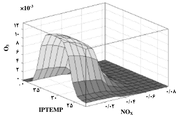
شکل ۶- بررسی اثر تغییرات غلظت ازون در مقابل تغییرات اکسیدهای نیتروژن و دمای هوا
