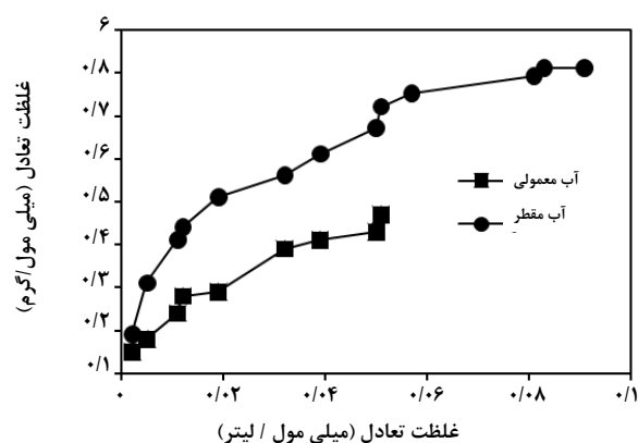
شکل ۵- تکدمای جذب کادمیم در آب مقطر و آب معمولی (میزان غلظت از ۰/۰۱۱ تا ۰/۳۸۷ میلی مول بر لیتر در آب مقطر و ۰/۰۰۹ تا ۰/۲۳۲ در آب معمولی، غلظت جلبک ۰/۰۹ میلی گرم بر لیتر)
