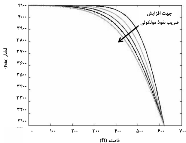
شکل ۱۱- تأثیر ضریب نفوذهای مختلف بر روی توزیع فشاری در زمان شبیه‌سازی ۲۰۰ روز و تراوانی ماتریس بلوک ۰/۰۱ md (در این شکل بیرونی‌ترین خط مربوط به حالتی است که ضریب نفوذ مولکولی ۰ (ft²/day) و خارجی‌ترین آن مربوط به حالتی است که ضریب نفوذ مولکولی ۲۰ (ft²/day) است. ضریب نفوذ مولکولی در بقیه خط‌ها به ترتیب از بیرونی به درونی ۵ (ft²/day)، ۱۰ (ft²/day) و ۱۵ (ft²/day) می‌باشند)
