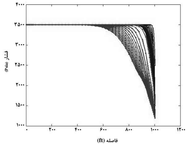
شکل ۳۶- توزیع فشاری با و بدون نفوذ مولکولی در ماتریس بلوک با تراوایی 0.0001 \text{ md} (در این شکل خط نقطه‌دار مربوط به حالتی است که در آن نفوذ مولکولی در نظر گرفته شده و خط بدون نقطه مربوط به حالت صرف نظر کردن آن می‌باشد)
