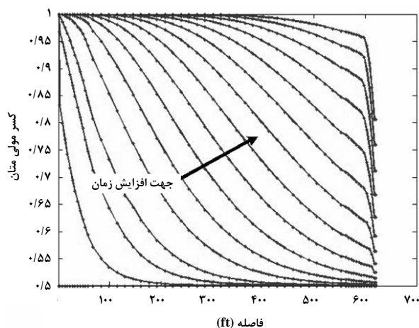
شکل ۱۰- توزیع کسر مولی متان برای ماتریس بلوک با تراوانی ۰/۰۱ md از زمان شبیه‌سازی ۳۰۰۰۰ روز تا ۱۰۰۰۰۰۰ با گام زمانی ۵۰۰۰۰ روز
