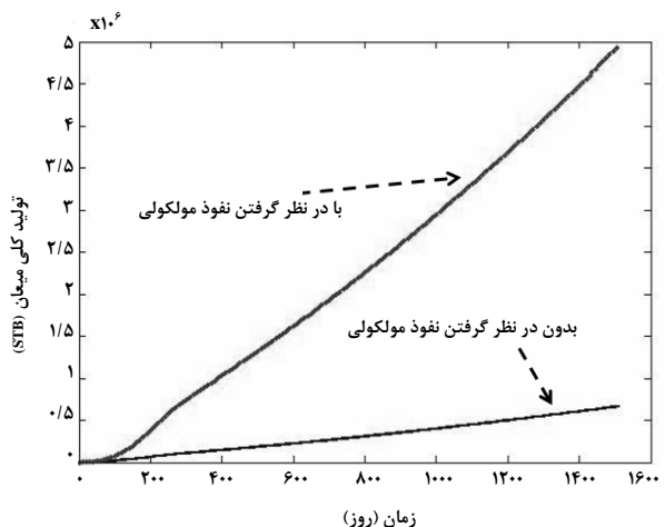
شکل ۳۹- تولید کلی میعانی با و بدون در نظر گرفتن نفوذ برای ماتریس بلوک با تراوایی 0.0001 \text{ md} (در این شکل خطوط با در نظر گرفتن نفوذ مولکولی و بدون در نظر گرفتن آن با پیکان نشان داده شده‌اند)
