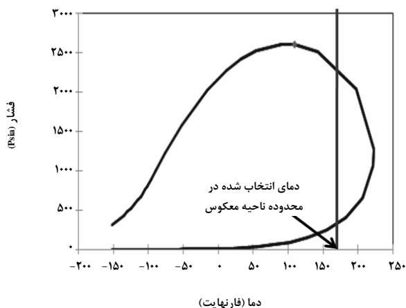
شکل ۲۲- نمودار فازي گاز میعانی سیال اشباع شده ماتریس بلوک و دمای در نظر گرفته شده
