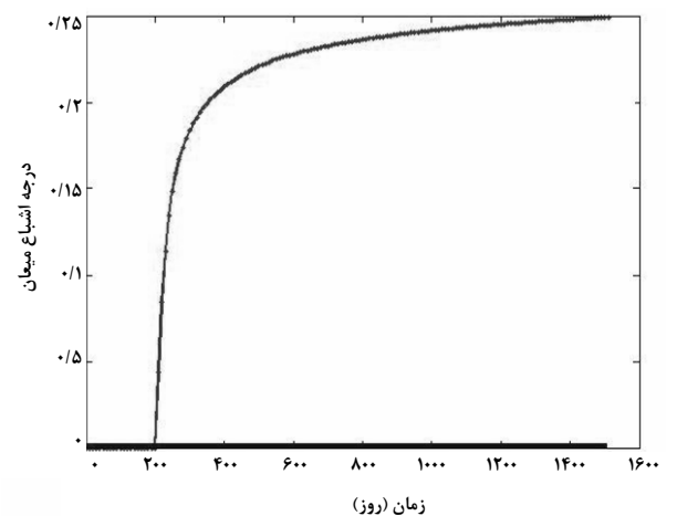
شکل ۳۷- درجه اشباع در شبکه بلوک 54 ، با و بدون در نظر گرفتن نفوذ برای ماتریس بلوک با تراوایی 0.0001 \text{ md} (در این شکل خطی که بر روی محور افقی واقع شده است مربوط به حالتی می‌باشد که در آن از نفوذ مولکولی صرف نظر شده و خط نقطه‌دار دیگر مربوط به حالتی است که در آن نفوذ مولکولی در نظر گرفته شده است)
