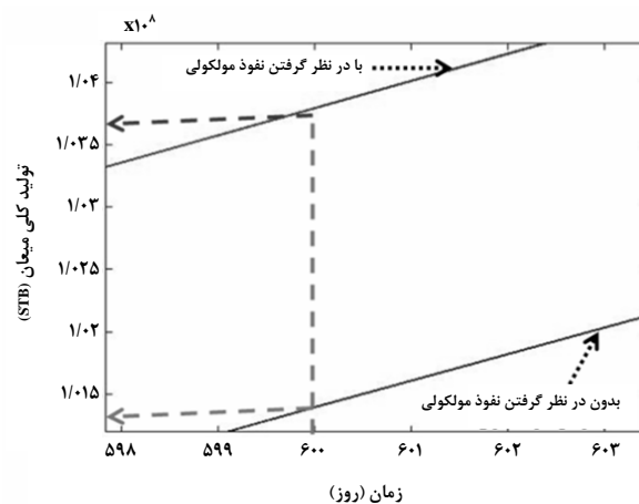
شکل ۳۳- تولید کلی میعان با و بدون در نظر گرفتن نفوذ مولکولی برای ماتریس بلوک با تراوایی 0.1 md، در یک زمان مشخص شبیه‌سازی (در این شکل خطوط با در نظر گرفتن نفوذ مولکولی و بدون در نظر گرفتن آن با پیکان نشان داده شده‌اند)
