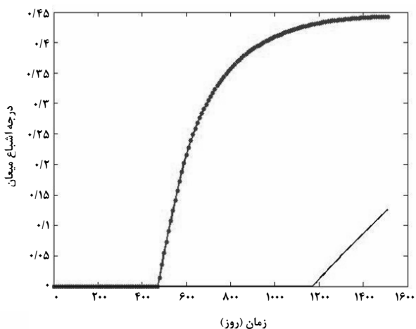
شکل ۳۱- درجه انشباع در شبکه بلوک 0.48 با و بدون در نظر گرفتن نفوذ برای ماتریس بلوک با تراوایی 0.001 md (در این شکل خط نقطه‌دار مربوط به حالتی است که در آن نفوذ مولکولی در نظر گرفته شده و خط بدون نقطه مربوط به حالت صرف نظر کردن آن می‌باشد)
