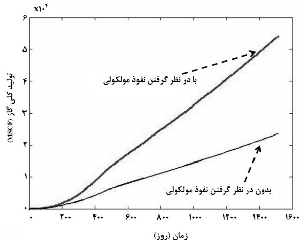
شکل ۳۴- تولید کلی گاز با و بدون در نظر گرفتن نفوذ برای ماتریس بلوک با تراوانی ۰/۰۰۱ md (در این شکل خطوط با در نظر گرفتن نفوذ مولکولی و بدون در نظر گرفتن آن با پیکان نشان داده شده‌اند)
