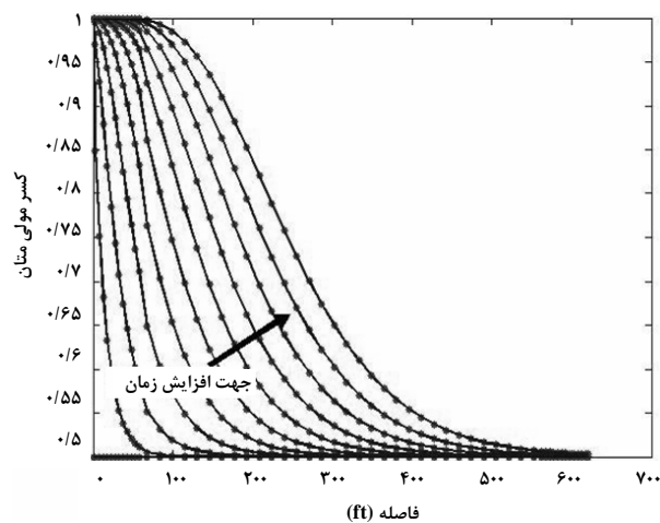
شکل ۱۲- کسر مولی متان با و بدون در نظر گرفتن نفوذ مولکولی برای ماتریس بلوک‌هایی با تراوایی ۱ md از زمان شبیه‌سازی ۱۰۰۰۰ روز تا ۱۰۰۰۰۰۰ روز و گام زمانی ۱۰۰۰۰ روز (در این شکل توزیع با در نظر گرفتن نفوذ مولکولی با خط نقطه‌دار نشان داده شده است که بر روی خط بدون در نظر گرفتن نفوذ مولکولی واقع شده است)
