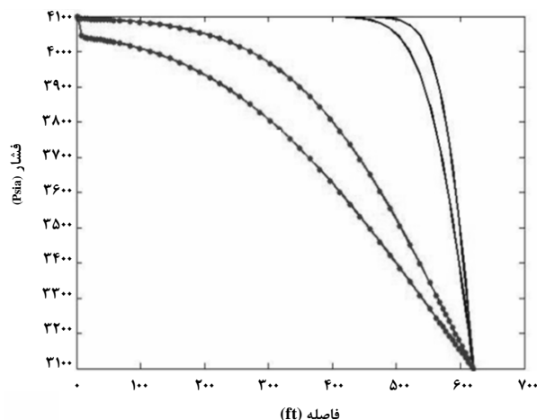
شکل ۱۷- توزیع فشار با و بدون در نظر گرفتن نفوذ مولکولی در حالت تراوانی ۰/۰۰۰۱ میلی‌داریسی، در زمان‌های ۱۰۰ و ۲۰۰ روز با گام ۱۰۰ روز (در این شکل خط نقطه‌دار مربوط به حالتی است که در آن نفوذ مولکولی در نظر گرفته شده و خط بدون نقطه مربوط به حالت صرف نظر نمودن آن می‌باشد)
