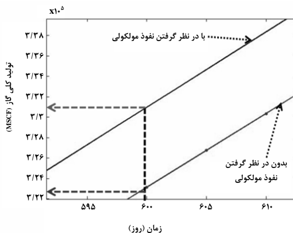
شکل ۳۲- تولید کلی گاز با و بدون در نظر گرفتن نفوذ مولکولی برای ماتریس بلوک با تراوایی 0.1 md، در یک زمان مشخص شبیه‌سازی (در این شکل خطوط با در نظر گرفتن نفوذ مولکولی و بدون در نظر گرفتن آن با پیکان نشان داده شده‌اند)
