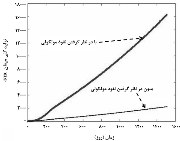
شکل ۳۸- تولید کلی گاز با و بدون در نظر گرفتن نفوذ برای ماتریس بلوک با تراوایی 0.0001 \text{ md} (در این شکل خطوط با در نظر گرفتن نفوذ مولکولی و بدون در نظر گرفتن آن با پیکان نشان داده شده‌اند)
