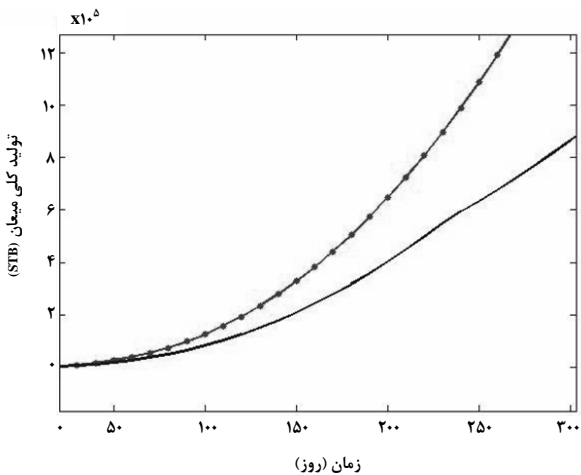
شکل ۳۳- تولید کلی میعان با و بدون در نظر گرفتن نفوذ برای ماتریس بلوک با تراوانی ۰/۰۰۱ md (در این شکل خطوط مربوط به حالتی است که در آن نفوذ مولکولی در نظر گرفته شده و خط بدون نقطه مربوط به حالت صرف نظر نمودن آن می‌باشد)
