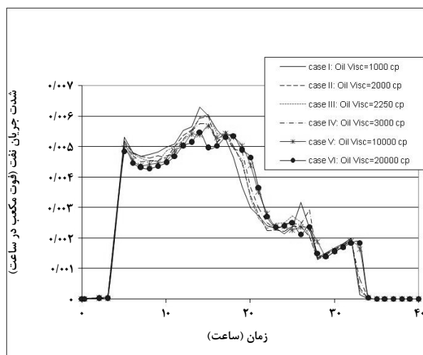
شکل ۱۴- اثر گرانروی اولیه نفت بر شدت جریان تولیدی در فرایند احتراق درجا
