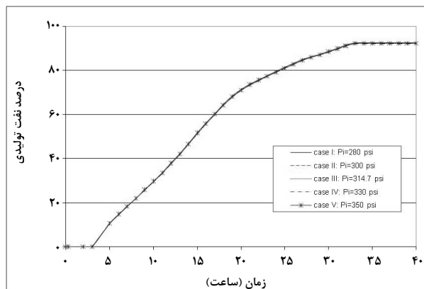
شکل ۱۵- اثر فشار اولیه بر درصد بازیافت نفت تولیدی
