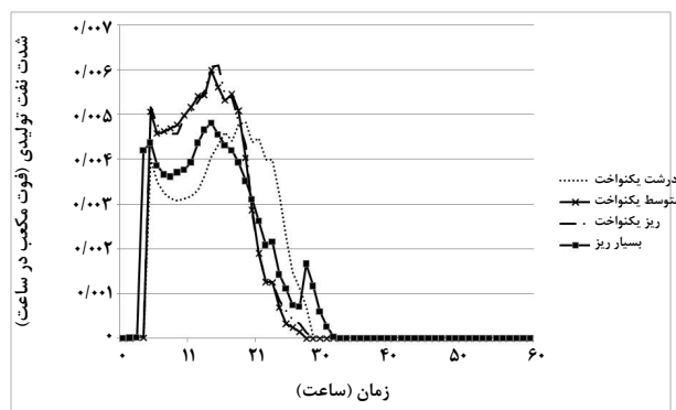
شکل ۲- اثر درجه‌بندی‌های مختلف بر شدت جریان تولیدی
