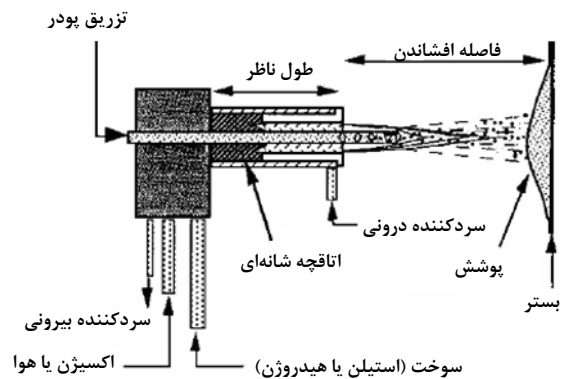
شکل ۱- دستگاه مورد استفاده برای افشاندن نانو ذرات سیلیس و CaCO 3 بر روی پلی آمیدها [۸].
