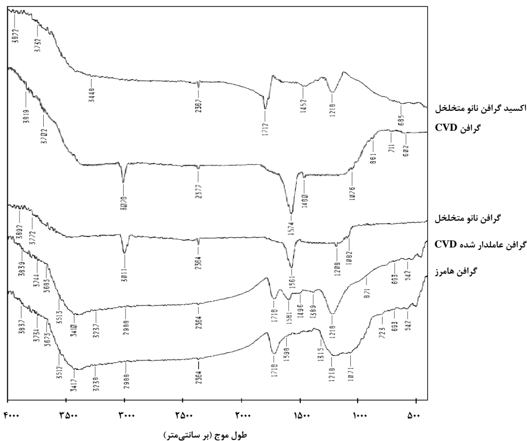
شکل ۳. طیف FTIR نانو ساختارهای گرافنی.
