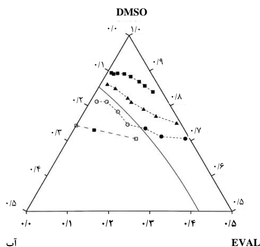
شکل ۱- دیاگرام فازی سیستم سه جزئی (آب/دی متیل) (سولفوکساید/پلی اتیلن-کو-وینیل الکل): (■) داده‌های تبلور در دمای ۲۵ درجه سلسیوس (-▲-) دمای ۴۵ درجه سلسیوس؛ (-●-) دمای ۶۵ درجه سلسیوس؛ (-○-) داده‌های باینودال در دمای ۶۵ درجه سلسیوس؛ (-) دمای ۲۵ درجه سلسیوس؛ (□-■-□) داده‌های تایلان [۹]
