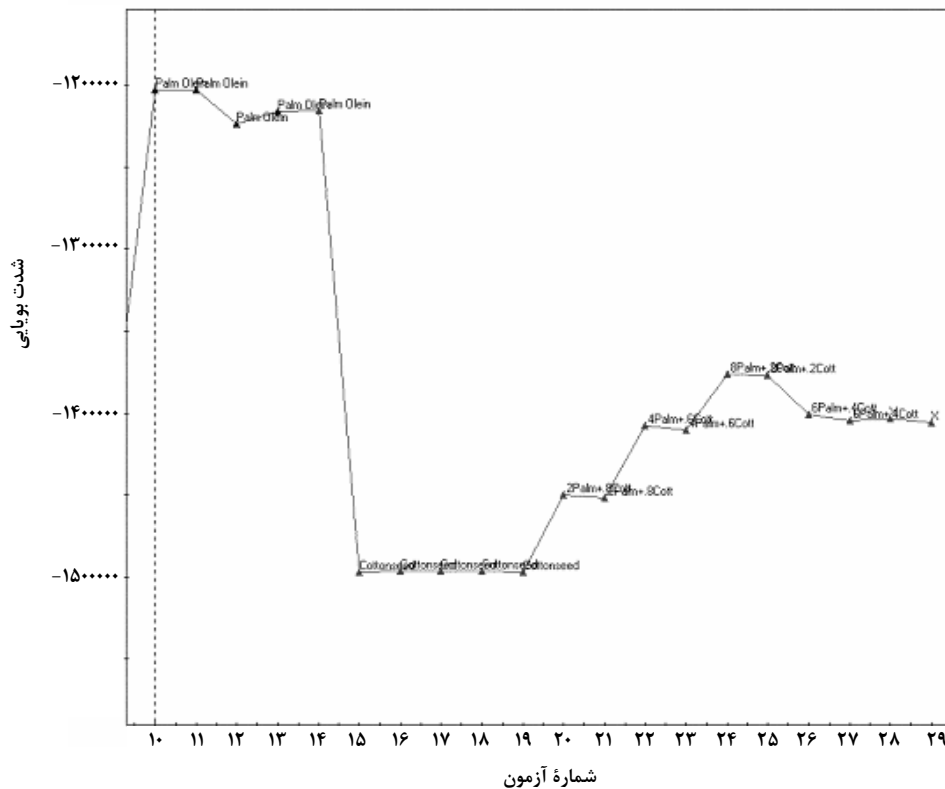
شکل ۳- نمودار کنترل کیفیت اماری روغن‌های پنبه دانه و پالم اولئین و مخلوط‌هایشان
